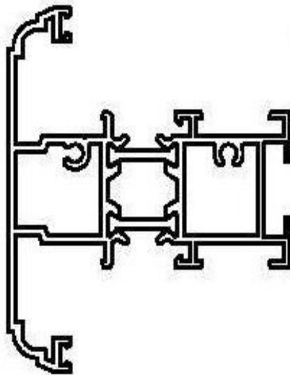
SWT 707 traverso anta
