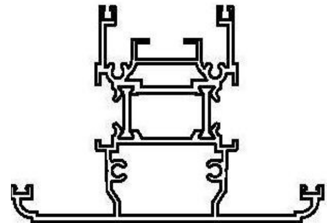
SW T708 traverso telaio
