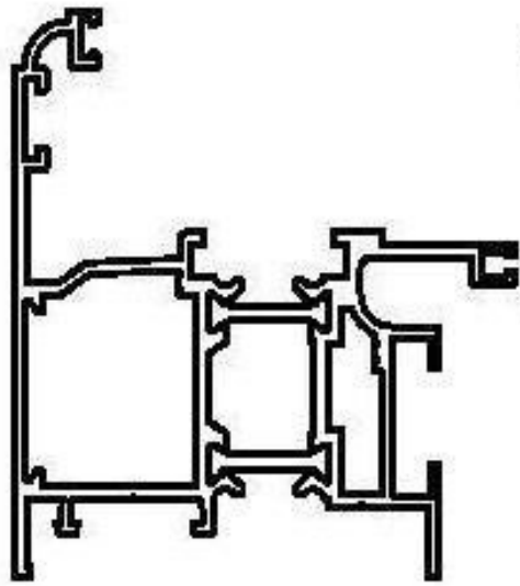
SW T701 telaio
