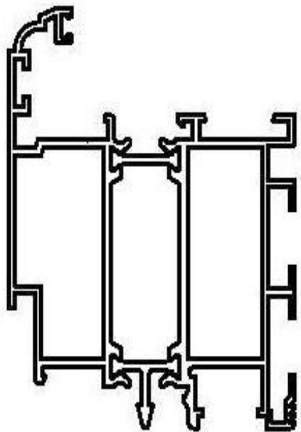
SW T705 anta maggiorata
